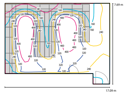
Lichtplanung (ISO-Linien zur Angabe der Beleuchtungsstärken in Lux an jedem Ort des Raumes)
